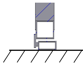
Tröskelanslag C-C SCALE 1 : 5
