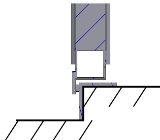
Anslag mot tröskeljern B-B SCALE 1 : 5
