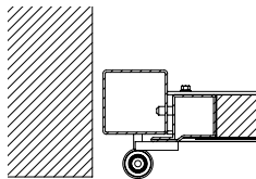
Slagport med rörkarm (Infälld)
