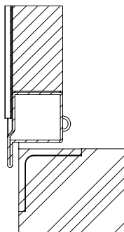
Anslag mot tröskeljärn B-B
