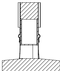
Släggummilist A-A
