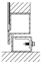
Tröskelanslag C-C
