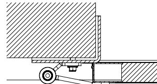
Slagport utanpåliggande
