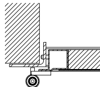
Slagport med L-karm (Infälld)
