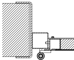
Slagport med U-ram (Infälld)
